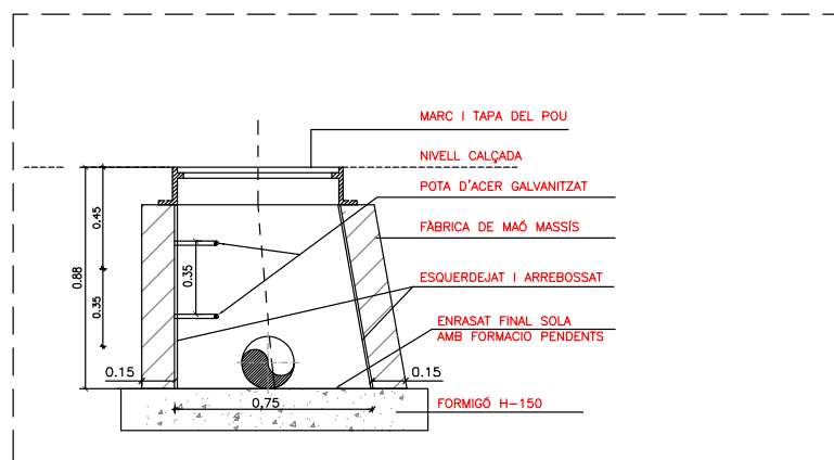
DETALL POU REGISTRE
