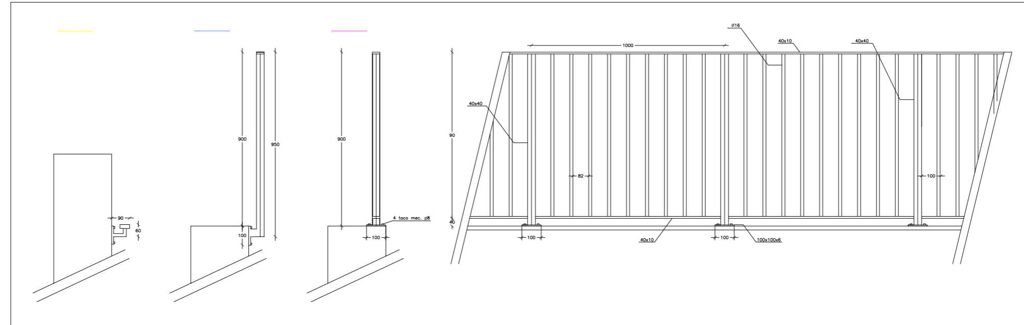
DETALL I ANCORATGE BARANES
