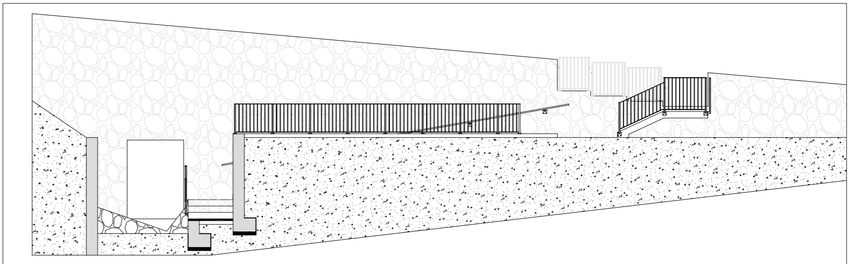
SECCIÓ B
